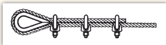
Montaggio corretto
