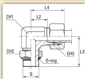
TIPO: EGC1061... ANELLO B3
