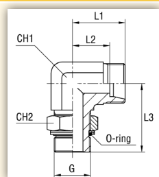
TIPO: EGC1061...1 SOLO CORPO
