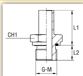
TIPO: EGC10CTG...M SOLO CORPO
