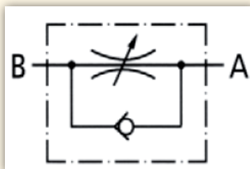
SCHEMA IDRAULICO
