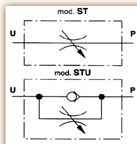
SCHEMA IDRAULICO
